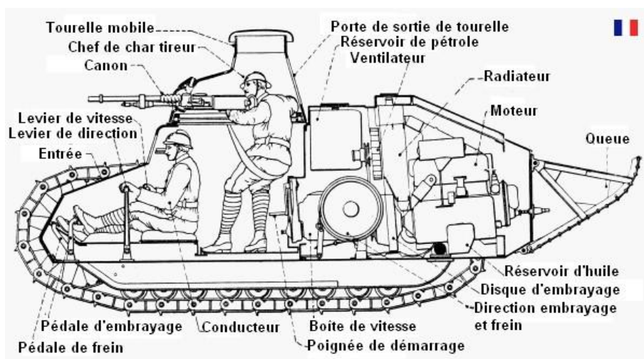
Char Renault FT-17 France diagramme de l'intérieur
